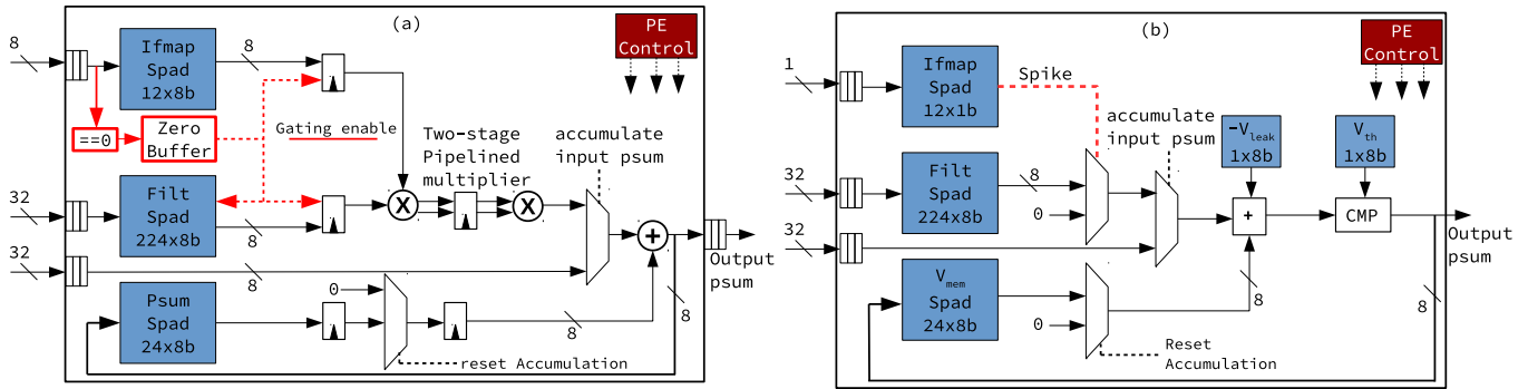
Fig. 3: (a) PE in Eyeriss [6]. (b) PE in Spiking-Eyeriss.
